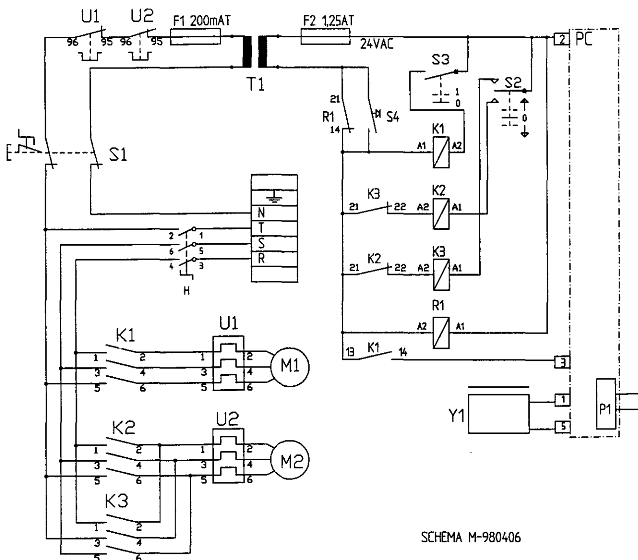
Fig. 3 Elschema för Sträckfilmsmaskin Manuell
